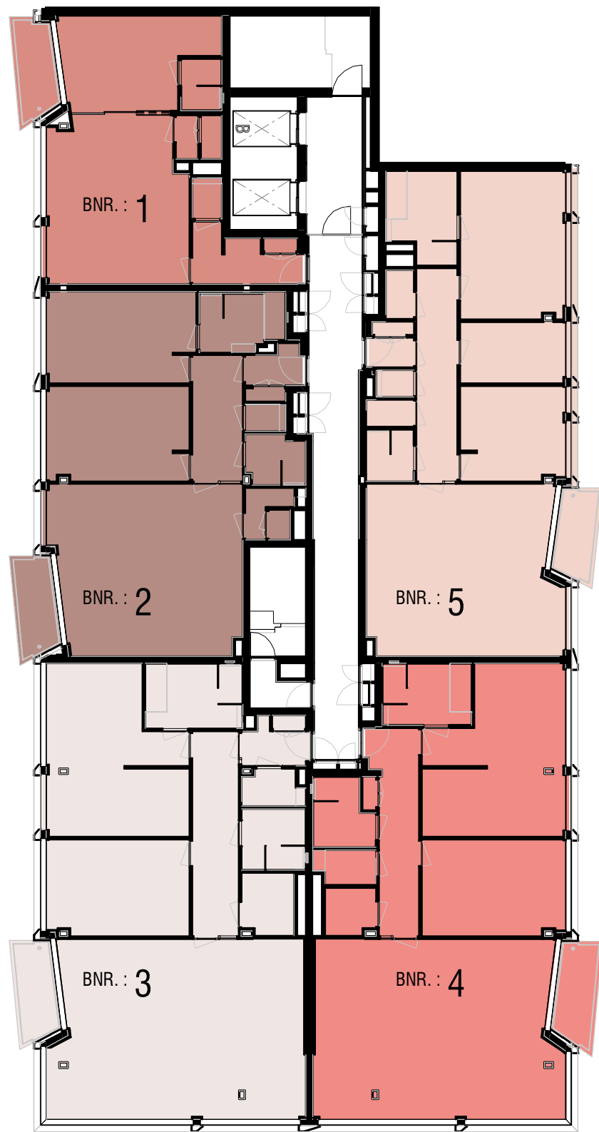
1 | 1ste verdieping (appartementen) 1 : 200
