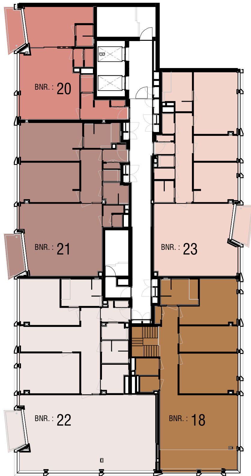
1 | 5de verdieping (appartementen) 1 : 200
