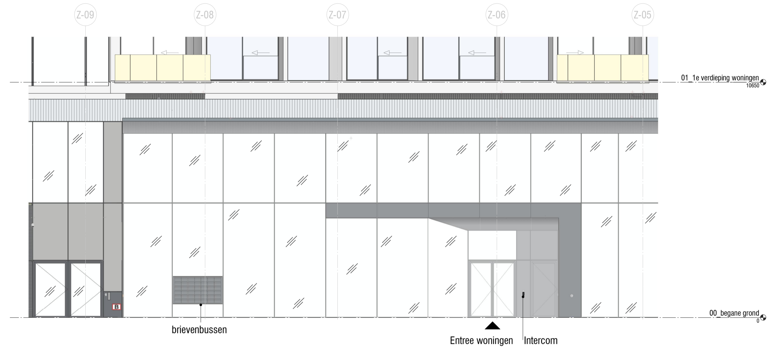
2 1:100 Aanzicht entree woningen WO.00-01.04-0002
